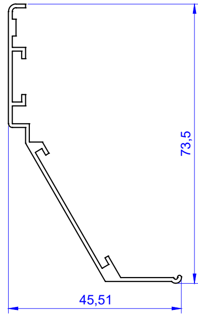
Profil No: 1085 Gramaj : 0.387 kg/m
