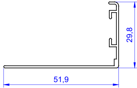
Profil No: 1074 Gramaj : 0.266 kg/m
