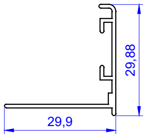
Profil No: 1086 Gramaj : 0.206 kg/m
