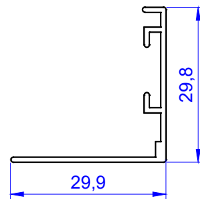
Profil No: 1087 Gramaj : 0.209 kg/m
