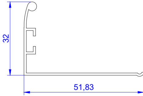
Profil No: 1073 Gramaj : 0.287 kg/m
