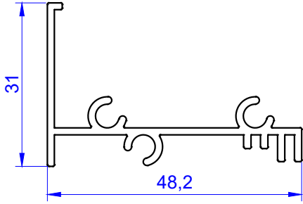
Profil No: 1088 Gramaj : 0.455 kg/m
