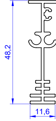
Profil No: 1089 Gramaj : 0.442 kg/m
